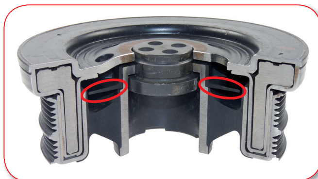
Abbildung 1: Torsionsschwingungsdämpfer mit Hitzeschutz
